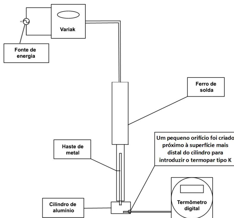
Figura 6 – Desenho esquemático do equipamento desenvolvido para a produção de queimaduras nos ratos
